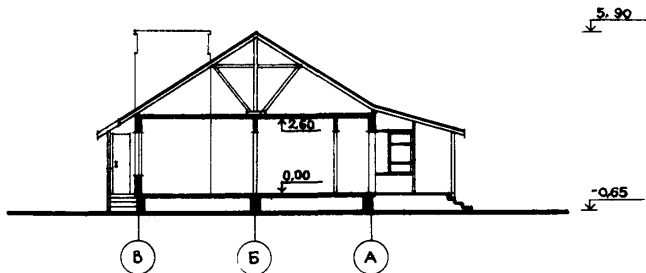
РАЗРЕЗ I-I
