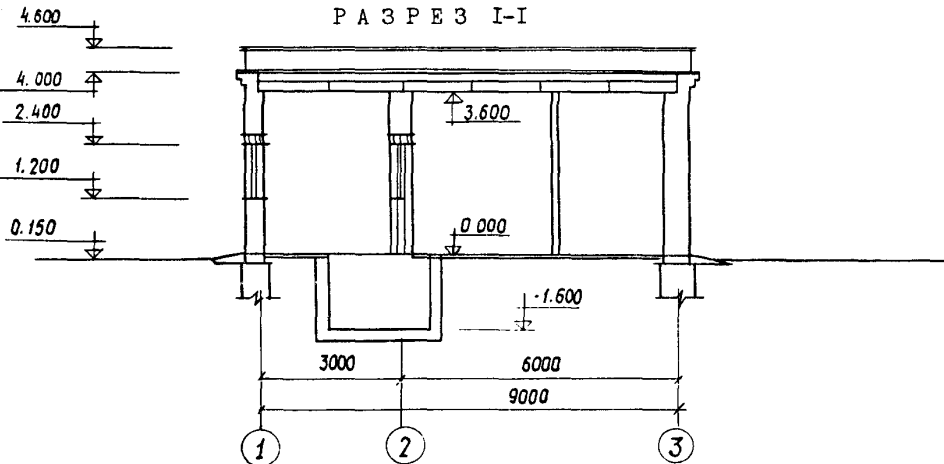
РАЗРЕЗ I-I
