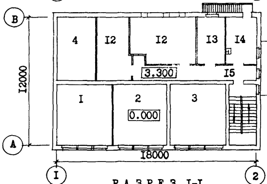
РАЗРЕЗ I-I
