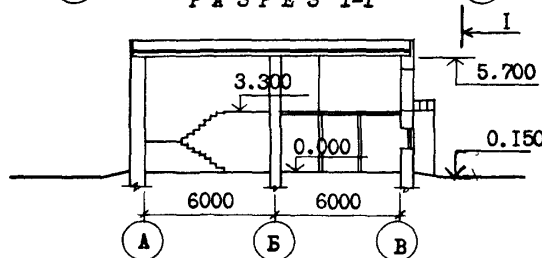
РАЗРЕЗ I-I
