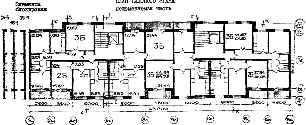
ЭКСПЛИКАЦИЯ КВАРТИР
