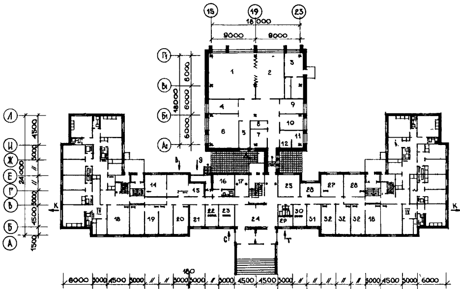
ПЛАН ТИПОВОГО ЭТАЖА
