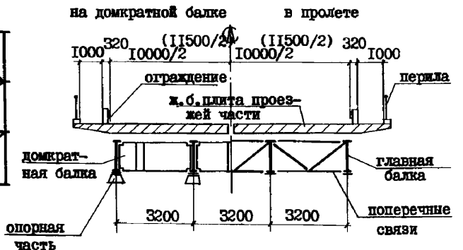
Поперечный разрез
