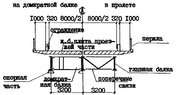
Поперечный разрез
