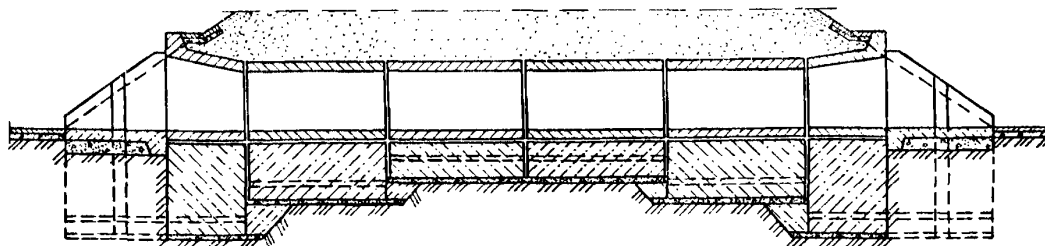
ТРУБА С ОГОЛОВКАМИ С ПАРАЛЛЕЛЬНЫМИ ОТКОСНЫМИ СТЕНКАМИ Продольный разрез
