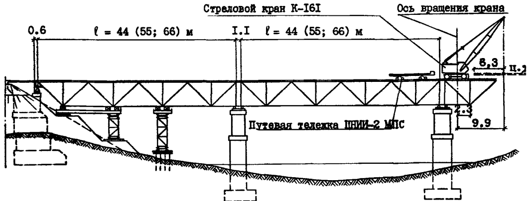
МОНТАЖ ПРОЛЕТНЫХ СТРОЕНИЙ l = 44, 55 \text{ и } 66 \text{ м} СТРЕЛОВЫМ КРАНОМ К-161
