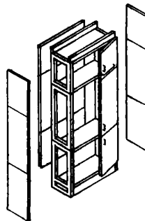
б) Встроенные шкафные отделения секций-перегородок h = 2,74 м под ригель
