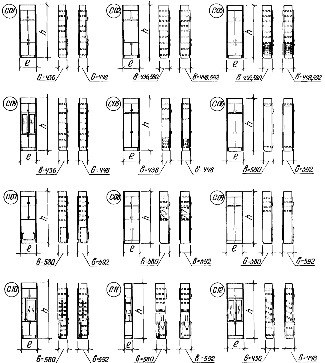
Эскизы секций со встроенными шкафными отделениями
