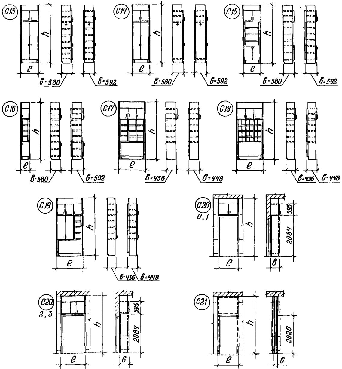
а) Встроенные шкафные отделения секций пристенных h=3,00 м под потолок
