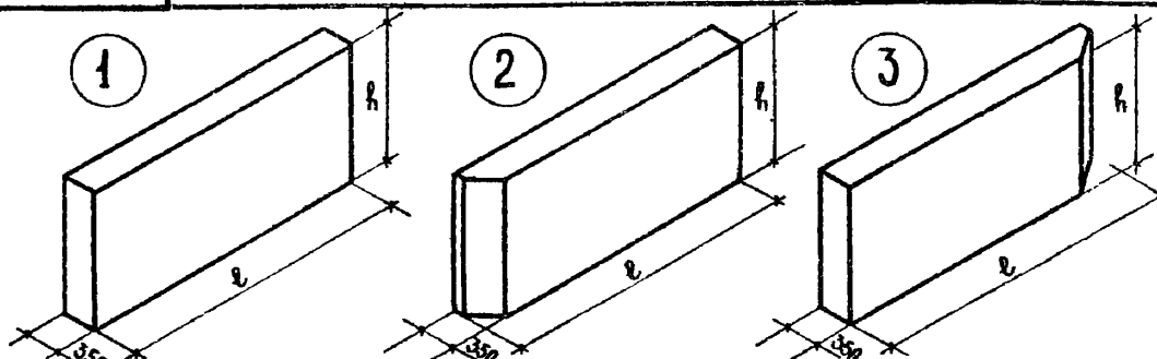
НОМЕНКЛАТУРА СТЕНОВЫХ ПАНЕЛЕЙ
