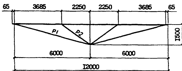
Схема прогонов типа ПР-, ПРС-
