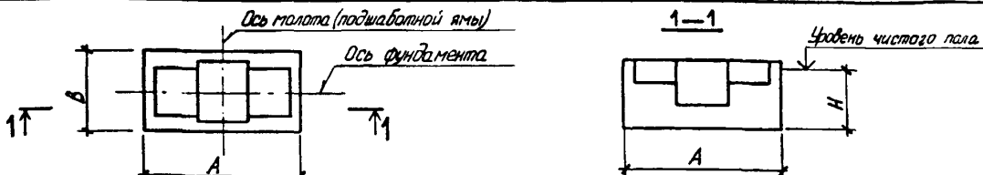
ТЕХНИЧЕСКИЕ ХАРАКТЕРИСТИКИ МОЛОТОВ И ГАБАРИТЫ ФУНДАМЕНТОВ
