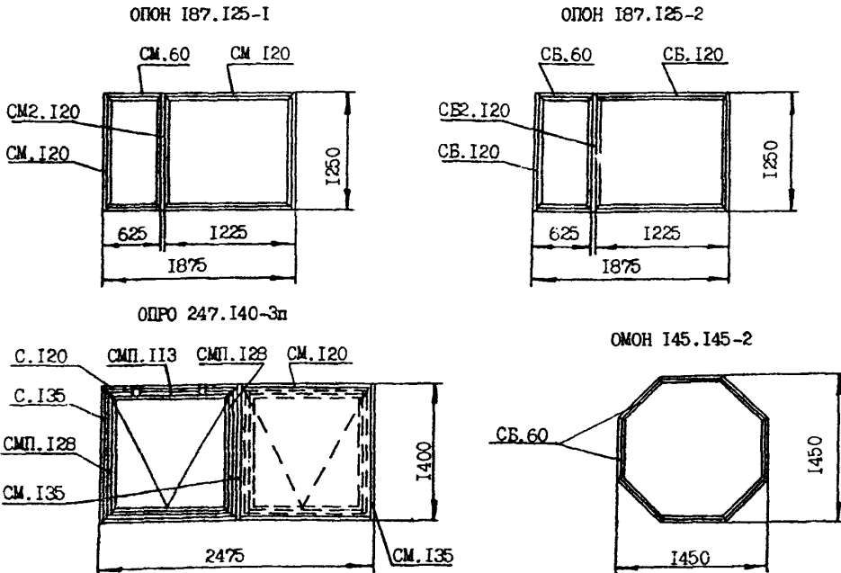
Примеры компоновки окон в зданиях
