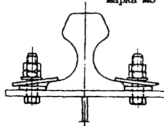
Крепление кранового рельса КР140 марка М3
