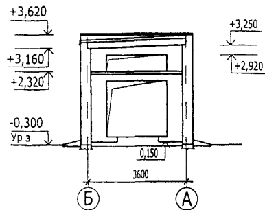
Разрез 1 - 1
