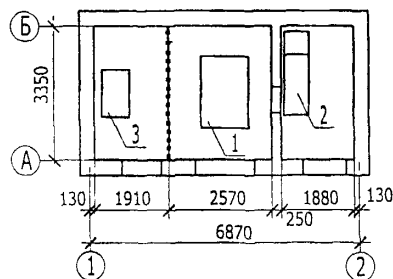
План расположения оборудования
