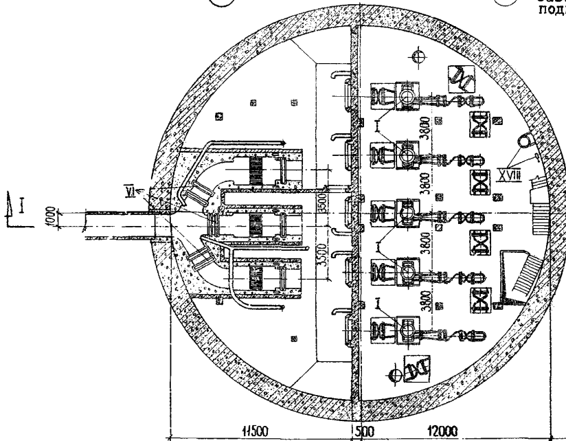
ПЛАН Б-Б
